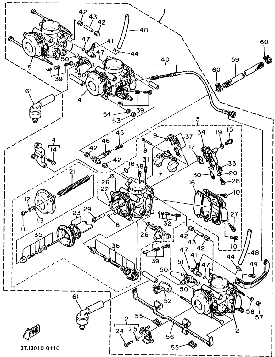
FIG. 11 キャブレタ 1 (3TJ1, 3TJ2)
