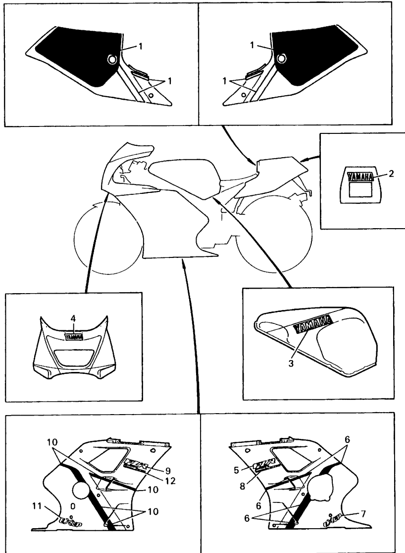
FIG. 53 グラフィック・エンブレム 2 (3TJ2)
