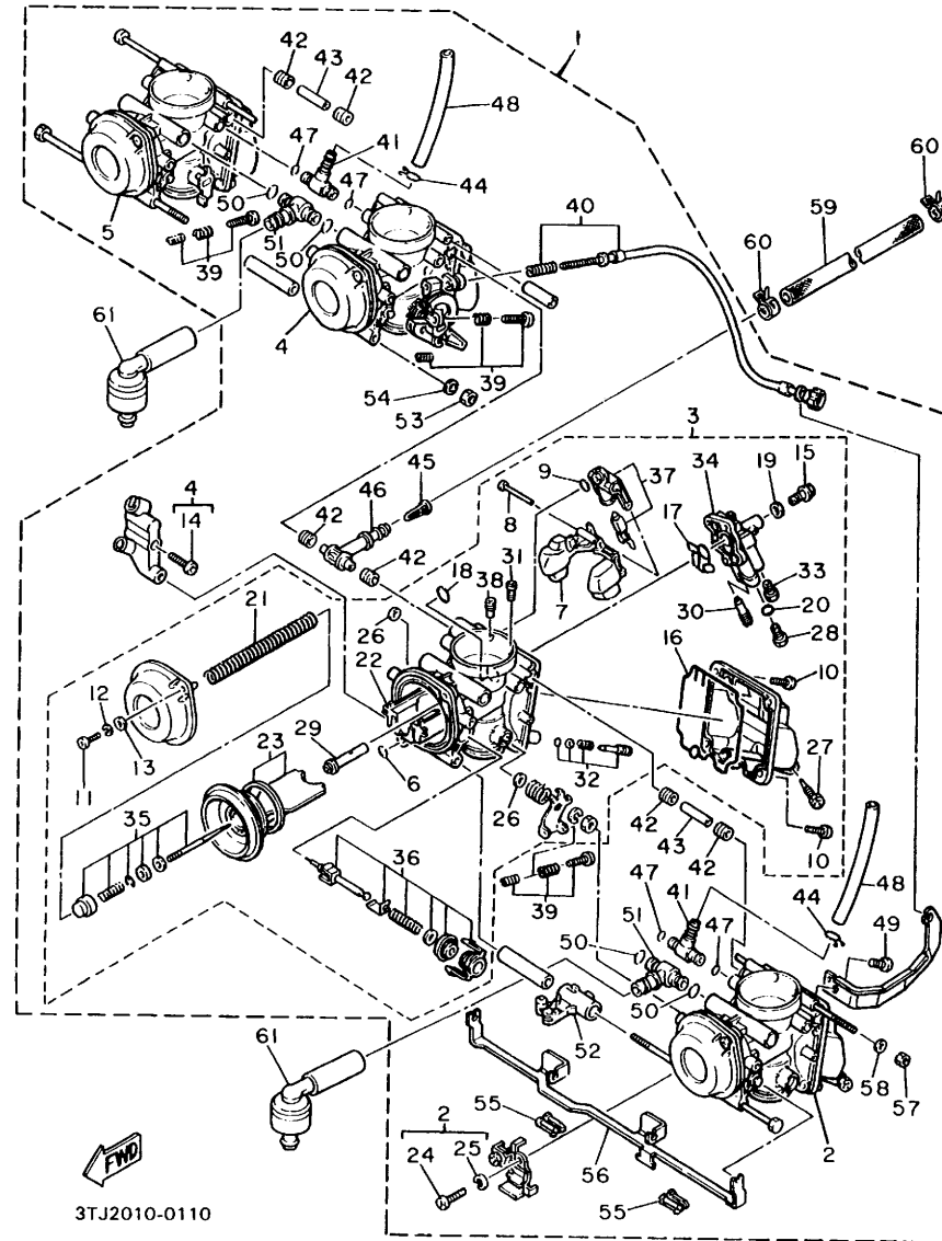
FIG. 11 キャブレタ 1 (3TJ1, 3TJ2)
