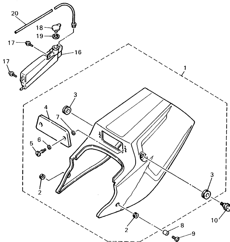
FIG. 26 サイドカバー 2 (3TJ2, 3TJ6, 3TJ7)
