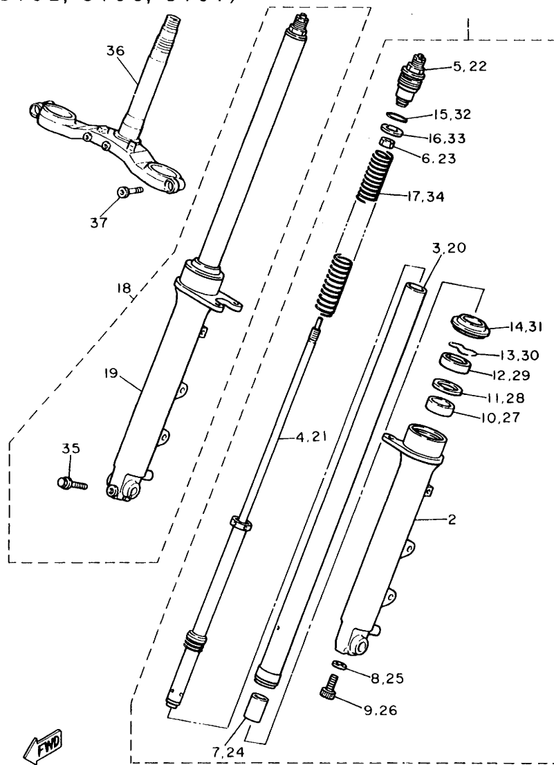
FIG. 31 フロントフォーク 2 (3TJ2, 3TJ6, 3TJ7)
